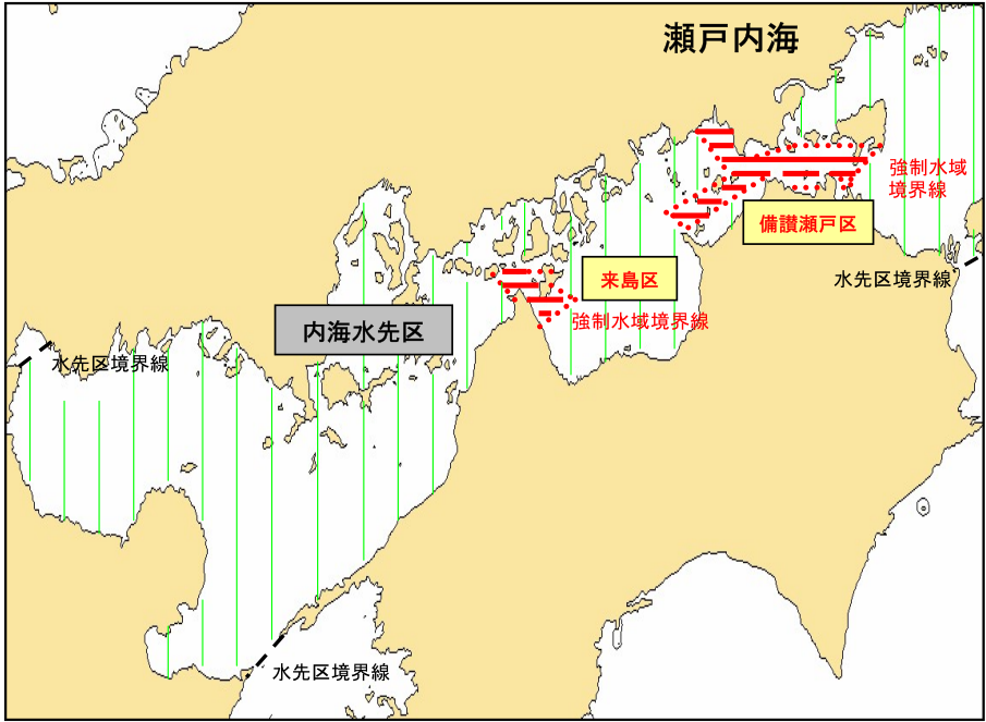
※ 強制水域は1万トン強制(備讃瀬戸区、来島区)
